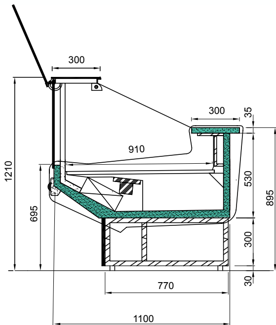
Libra EV-P
