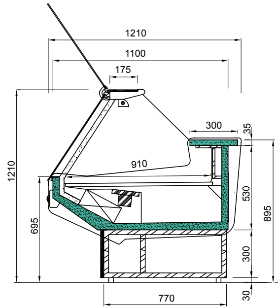
Libra EV-P
