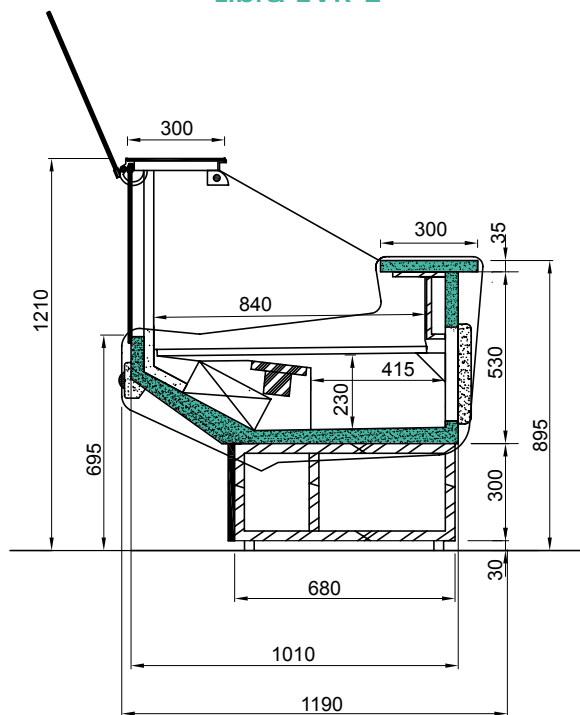
Libra EVR-2
