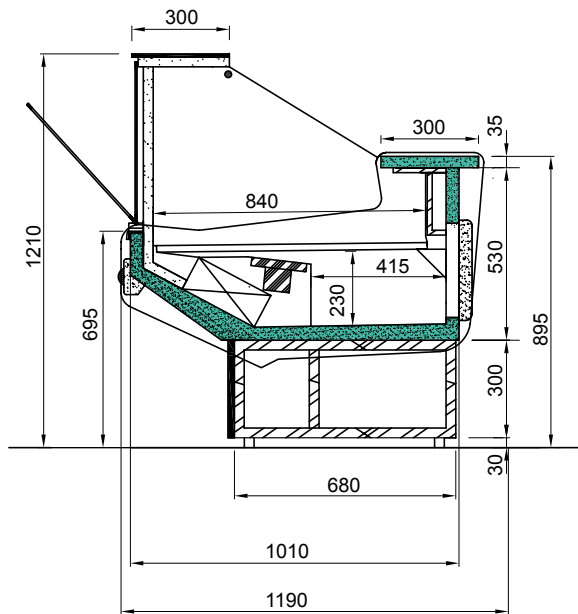
Libra EVR-2
