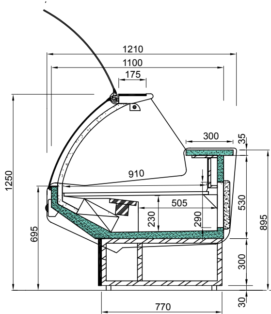
Libra EVR-P
