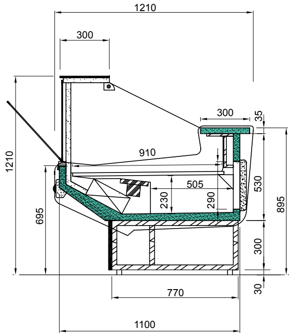
Libra EVR-P
